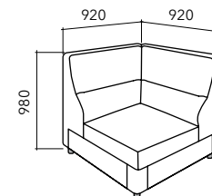
Секция угловая (взаимозаменяемая)
