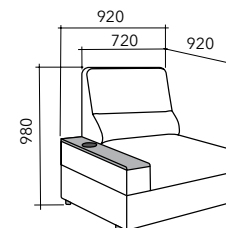
Секция угловая с полкой (правая, левая)
